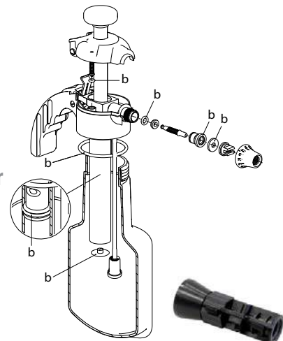
Foam nozzle G3/8"
